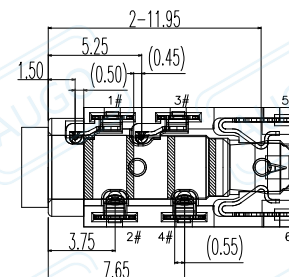
5极插头接触点位置尺寸
