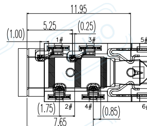
4极插头接触点位置尺寸
