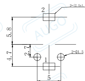
P.C.B 布局 焊料俯视图
